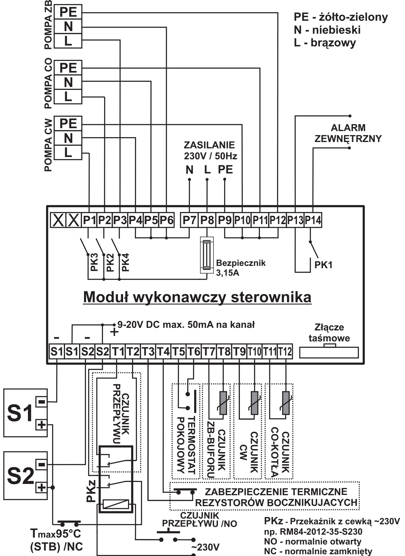
Schemat 1. Przykład podłączenia elementów wykonawczych i czujników do modułu wykonawczego z uwzględnieniem dodatkowych zabezpieczeń.
